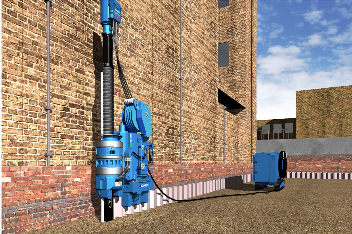
硬質地盤対応ゼロパイラーによる施工イメージ図
