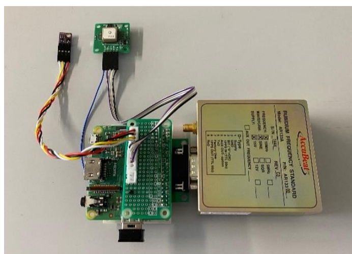
原子時計を使用したIoT(Internet of Things)システムの試作機
