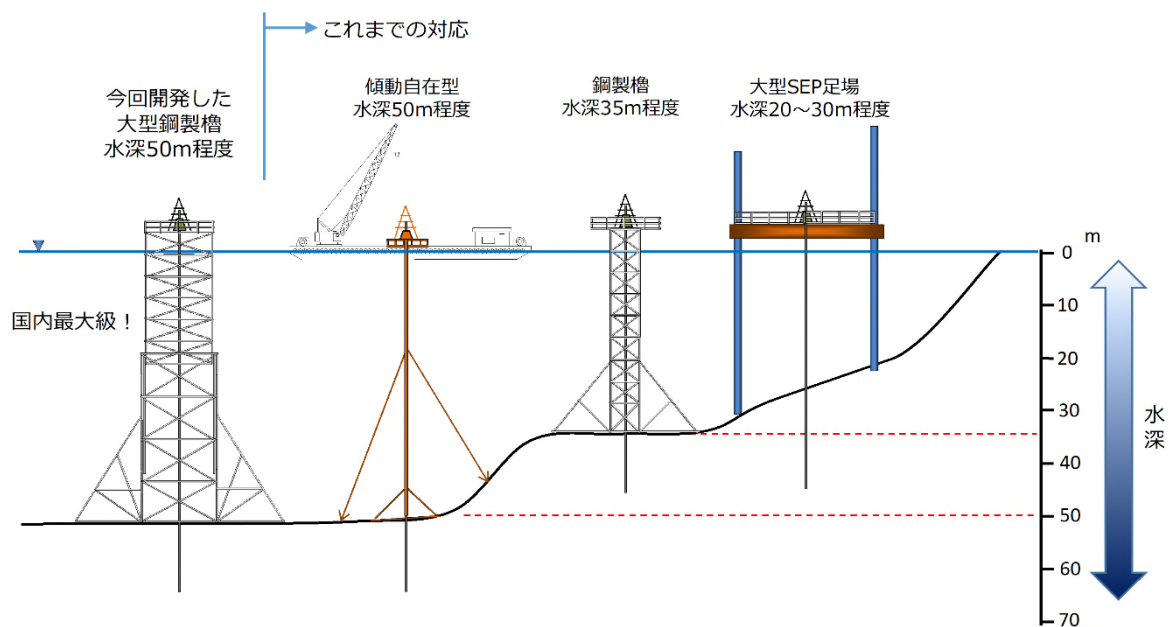
図 1 調査に用いられる仮設構造物
