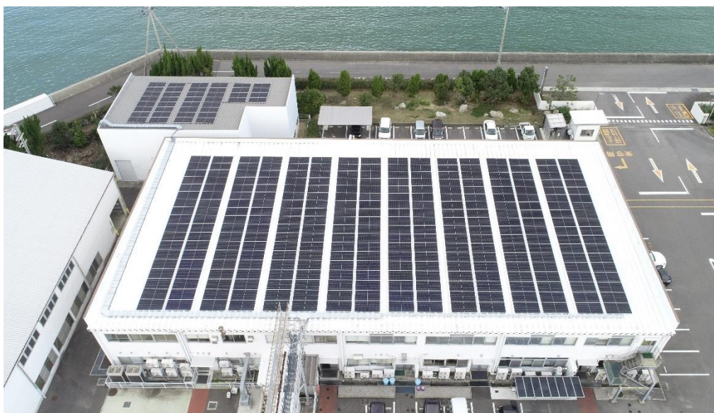
南海プライウッド 志度工場 太陽光発電システム
